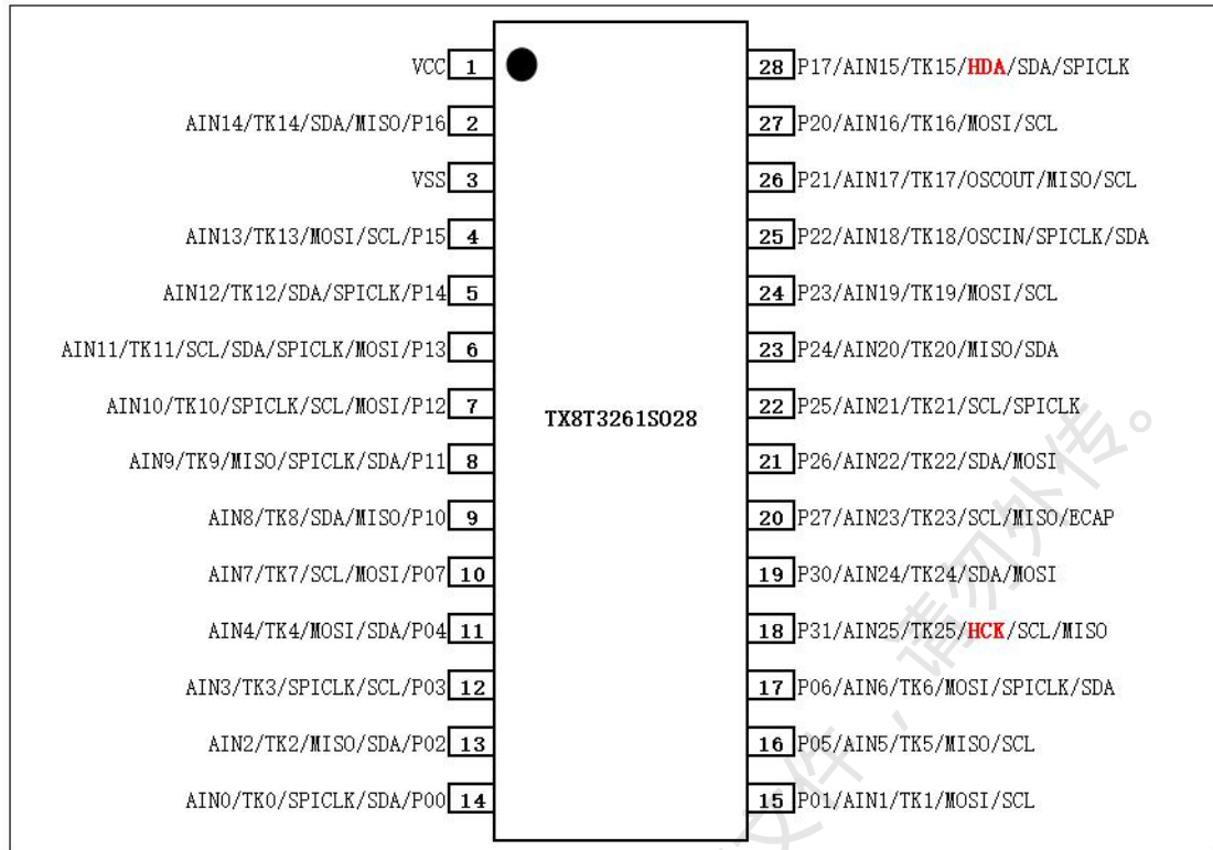
图 3 - TX8T3261S028 (SOP28) 封装图
